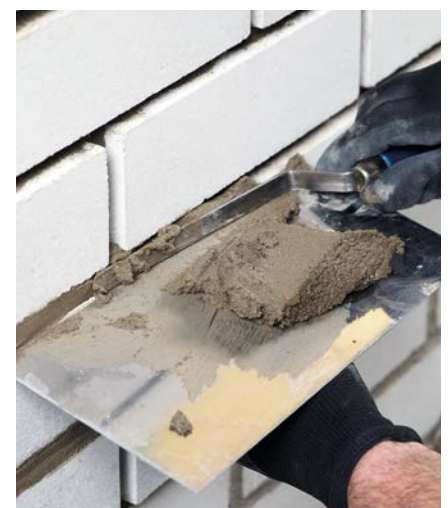
Bild 8 Nachträgliche Verfugung
