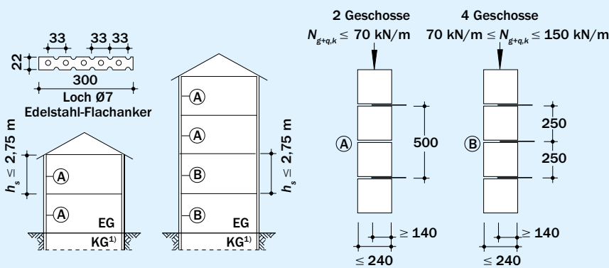
Bild 38 KS-Stumpfstoßtechnik, Regelausführung bei Annahme einer drei- oder vierseitigen Halterung der tragenden Wand (Schichthöhe \leq 25 cm) [3]
