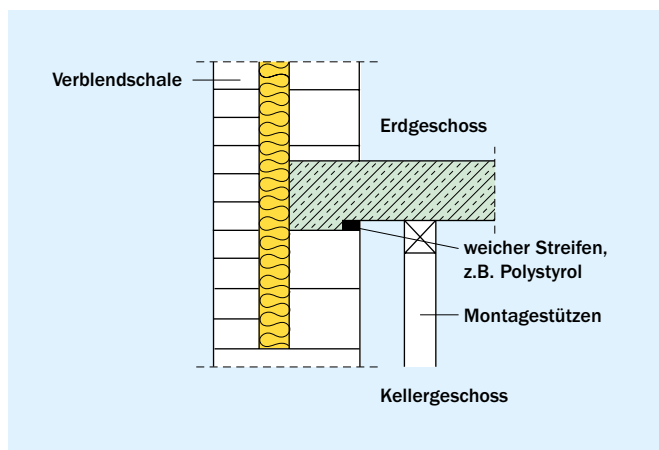
Bild 31 Konstruktive Zentrierung
