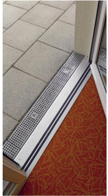
Bild 28: Schwellenfreier Übergang mit Lochblechabdeckung
